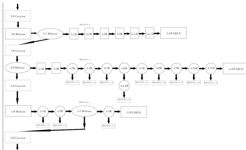
Figura 4.2. A árvore de versões (release) do FreeBSD
